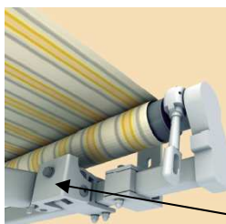
Uchwyt ramion ze śrubą regulacyjną
